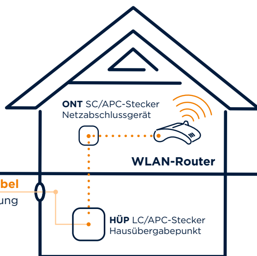
Verlegebeispiel
